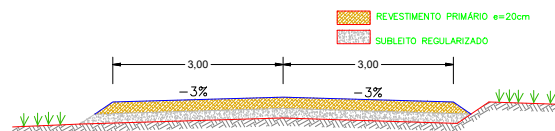
SEÇÃO TIPO DO REVESTIMENTO PRIMÁRIO e=20cm S/ ESCALA TODOS OS TRECHOS
